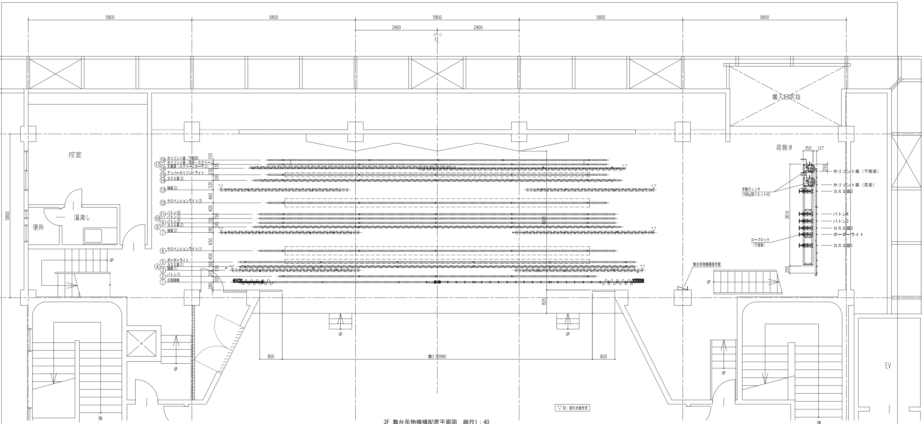
3F 舞台吊物機構配置平面図 縮尺1:40
